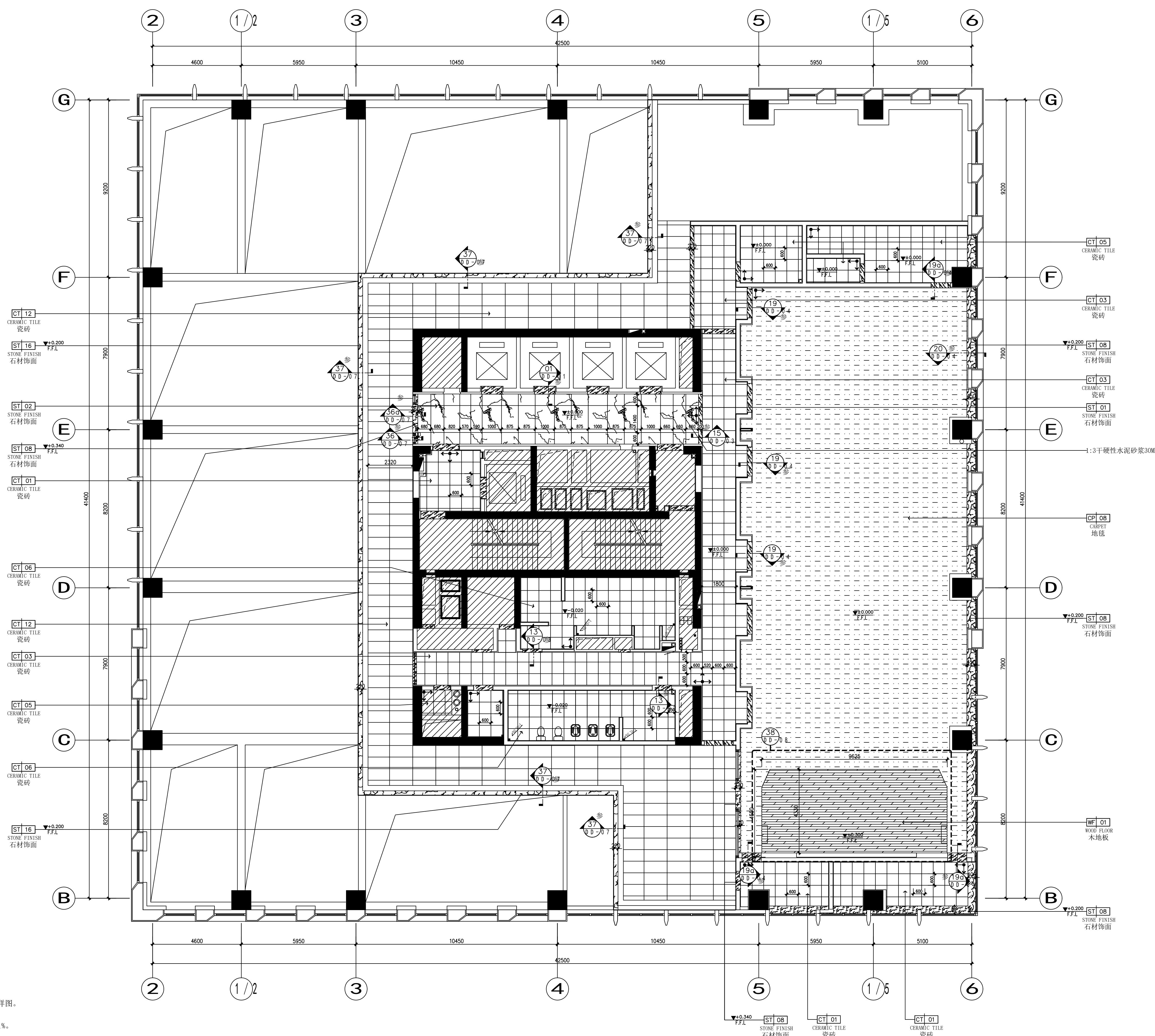
3 2 层地面铺装图 SCALE: 1:100 FLOOR MATERIAL PLAN
